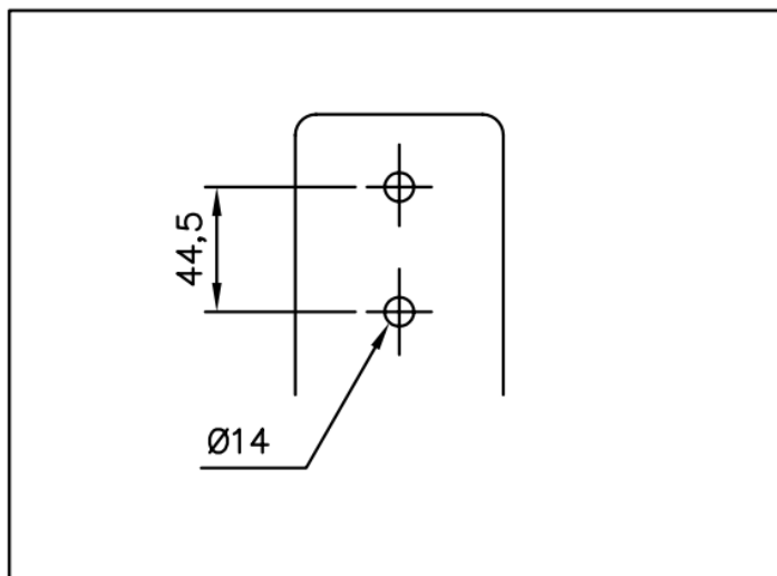
Figura 1 - furação dos terminais de alta tensão
